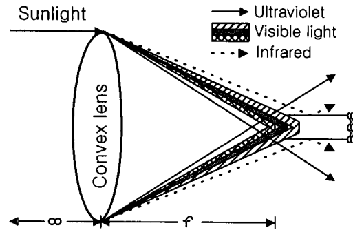
그림 2. 색수차를 이용한 태양광의 분리 Fig. 2. Spectral zone selection utilizing chromatic aberration
