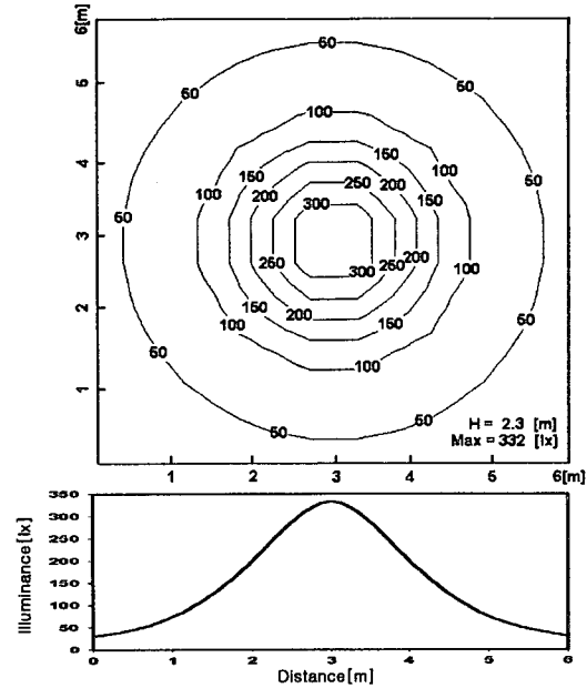
그림 7. 6가닥 한묶음 광섬유 채광시스템에 대한 작업면의 조도분포 시뮬레이션 Fig. 7. Simulation of illuminance pattern on the work-plane for a sunlight collector system comprised of a bundle of six core optical fibers
