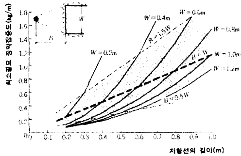
그림 4. 최소저항선 거리와 자유면의 크기에 따른 장약집중도
