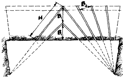
그림 1. 보조심발공을 배치한 V-cut 발파
