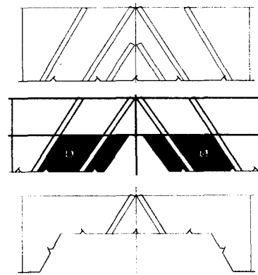
① V-cut 발파 천공배열 ② 보조심발공 발파후 ③ 자유면이 큰 심발발파
