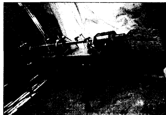
그림 10. 미국 유타대학교의 고속카메라 및 SHB 실험장치
