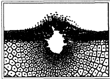
그림 17. 개별요소법을 이용한 cratering 모델링
