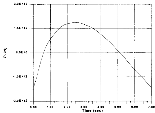
그림 15. 폭원하중의 시간이력곡선
