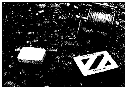
그림 13. 한국지질자원연구원의 고속촬영 시스템과 다단발파기
