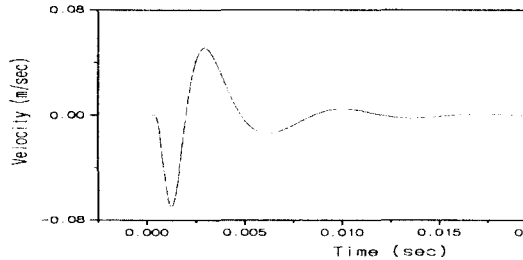
그림 16. FLAC으로 계산한 20m 지점에서의 진동 파형
