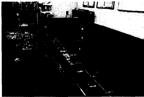
그림 6. Split Hopkinson Bar를 이용한 동적 실험 장치
