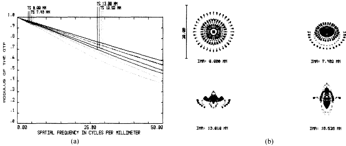
그림 5. 광학성능.
