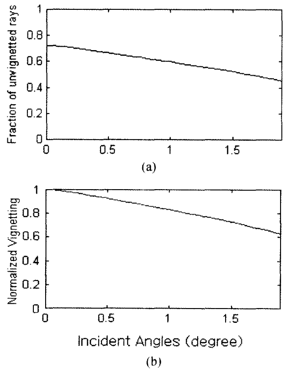
그림 7. Normalized 비축광량차폐(Vignetting).
