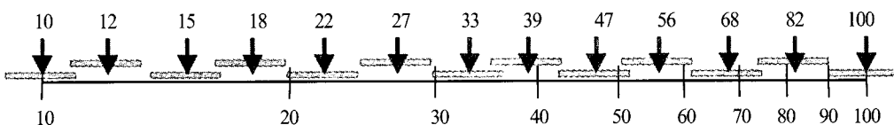
그림 2. 10% 저항의 공칭값과 실제 저항값의 범위
