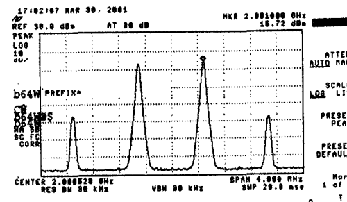
그림 4. PBG 와 CPW를 이용한 증폭기 IMD 특성
