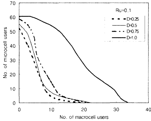
그림 9. 마이크로셀의 위치에 따른 용량 평면도(Ru=0.1)
