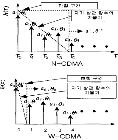
그림 3. 대역폭에 따른 N-CDMA와 W-CDMA의 다중 경로의 영향 (제한한 방법).
