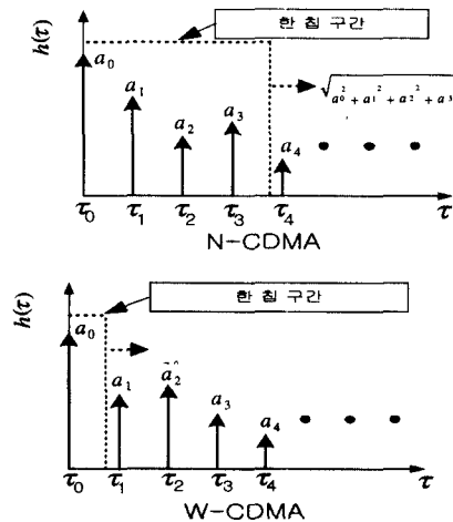
그림 2. 대역폭에 따른 N-CDMA와 W-CDMA의 다중 경로의 영향 (기존의 방법).
