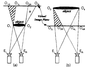
그림 2. 스테레오 영상에서 폐색 영역의 위치
