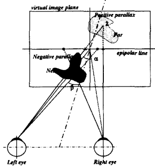
그림 8. 수평 시차
