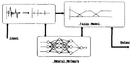
그림 5. Neuro-Fuzzy Diagnosis Model
