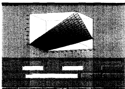
그림 10. 학습결과 얻어진 진단모델의 Surface 분포도
