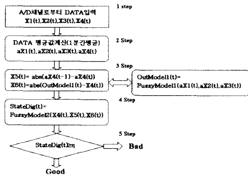
그림 6. 진단알고리즘의 흐름도
