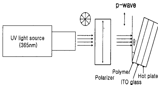
그림 2. UV 조사 시스템.
