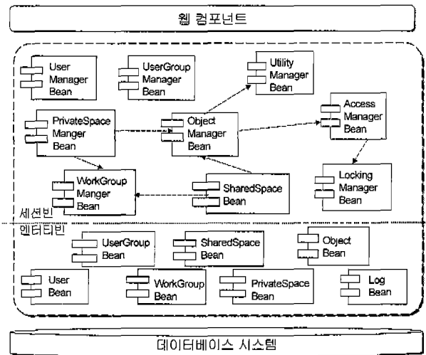
(그림 3) iPlace 시스템의 협업지원 컴포넌트 구조
