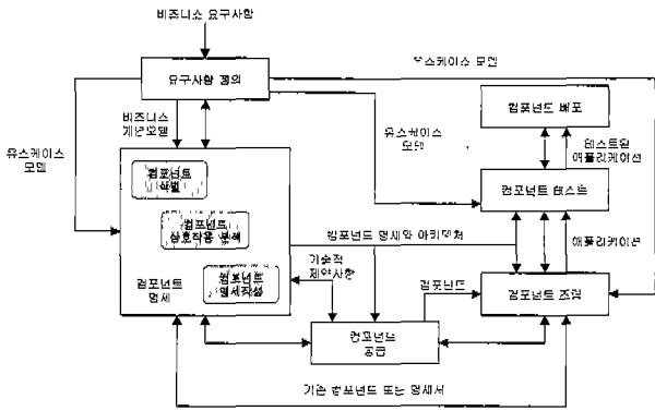
(그림 9) IDAO의 구현 프로세스 워크플로우
