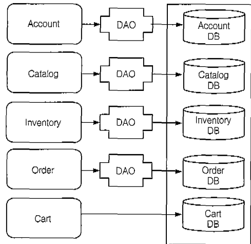
(그림 2) 레거시 시스템에서의 DAO 구조도
