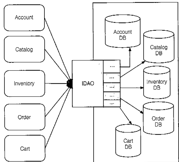
(그림 8) Iterator 패턴을 적용한 IDAO
