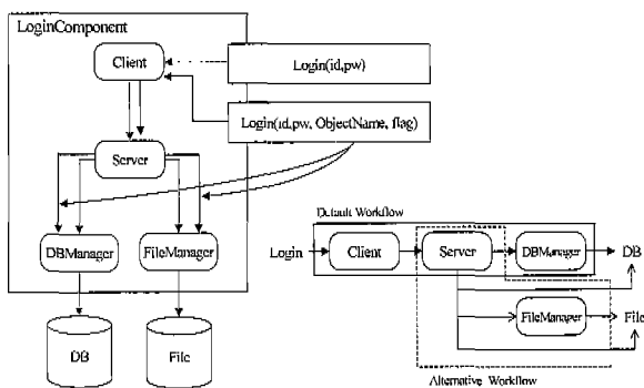
(그림 4) 사용자 인증 컴포넌트
