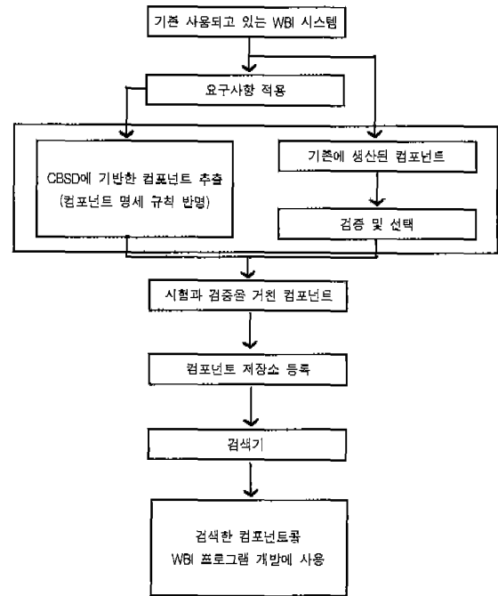
(그림 2) 제안 시스템 순차도
