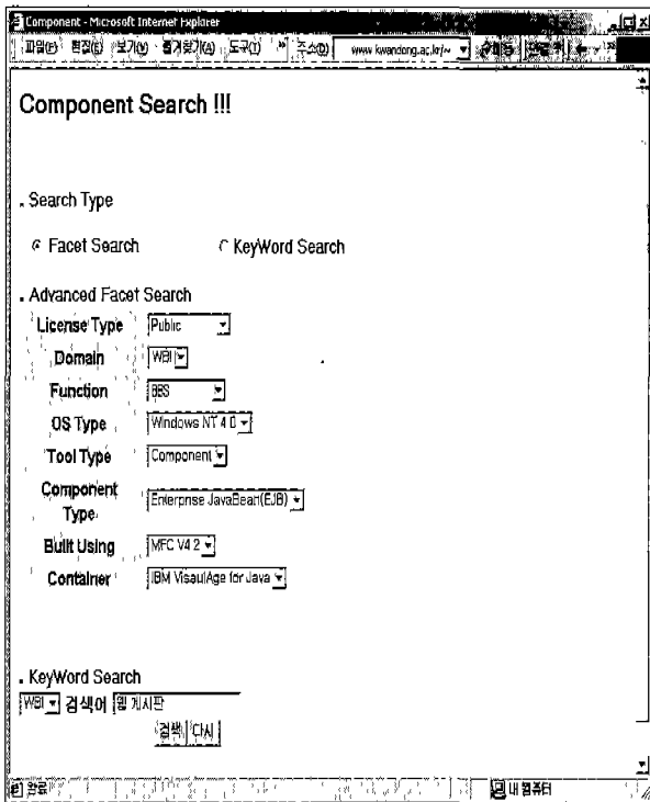
(그림 10)컴포넌트 검색 화면
