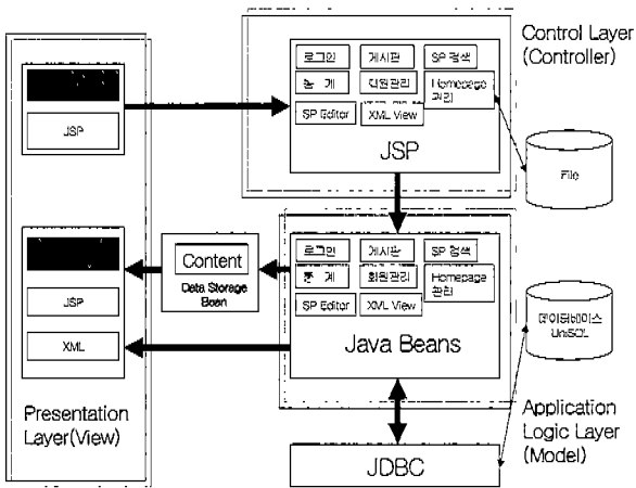
(그림 4) 표준프로파일 관리시스템 아키텍처
