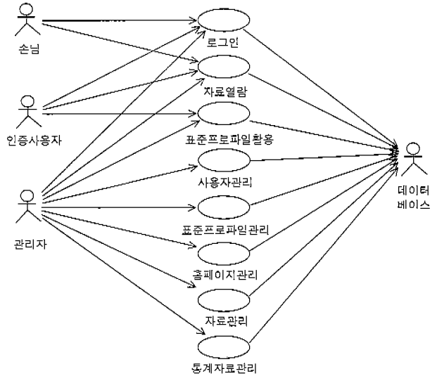
(그림 5) 표준프로파일 관리시스템 UseCase Diagram
