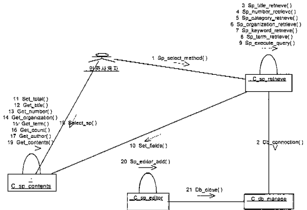
(그림 10) 개별프로파일 선택 지원도구 기능 중 표준프로파일 추가 기능에 대한 협동 다이어그램
