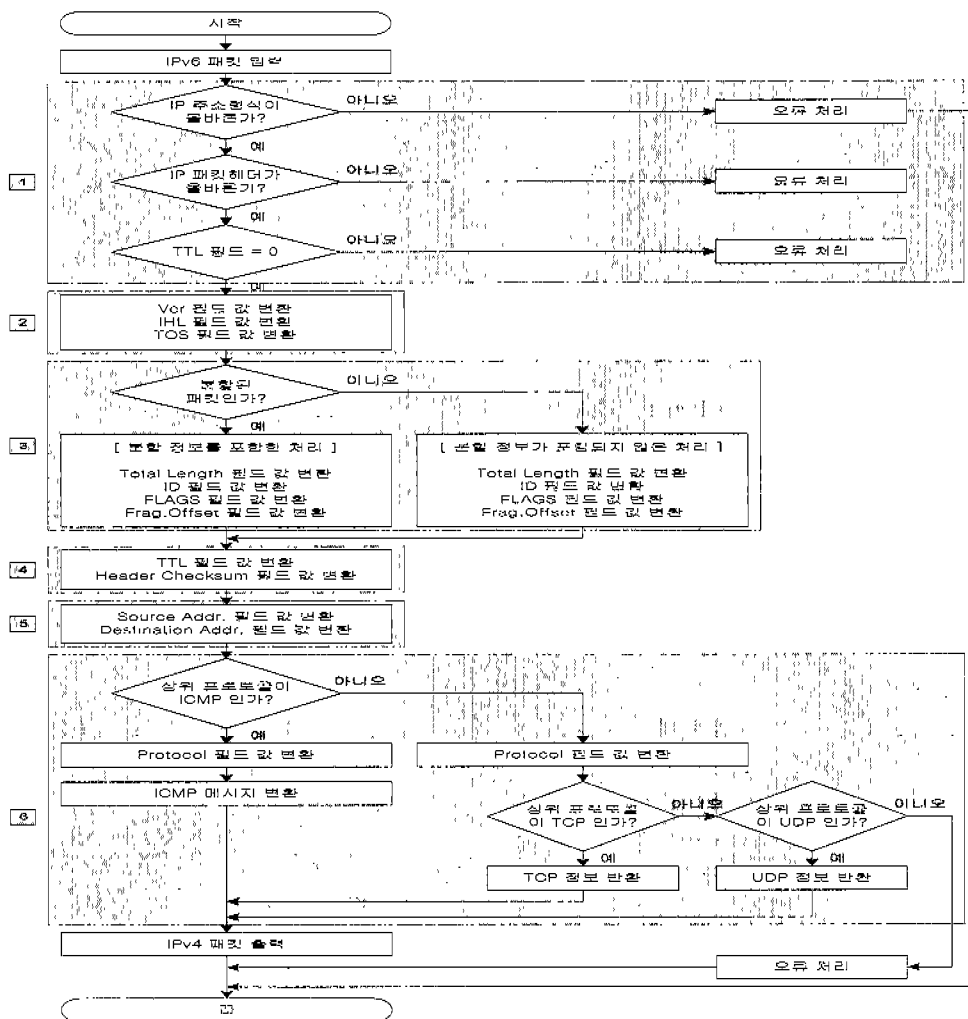
(그림 8) IPv6-to-IPv4 프로토콜 변환 기능부의 동작 절차
