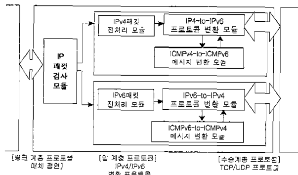
(그림 10) IPv4/IPv6 변환 프로토콜의 기능 모듈구조
