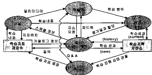
(그림 2) CSMA 학습시스템 모델
