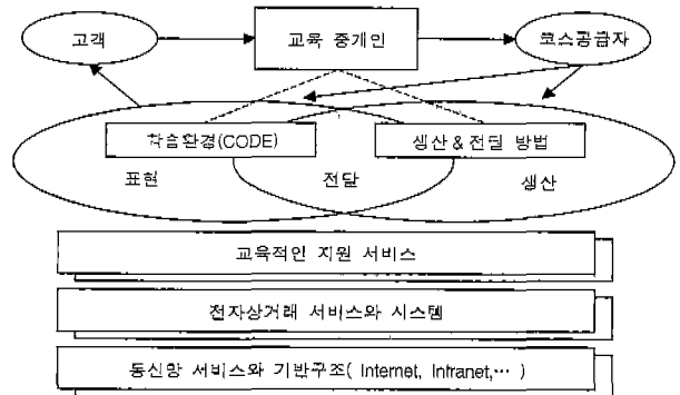
(그림 1) CODE의 시스템 구조도
