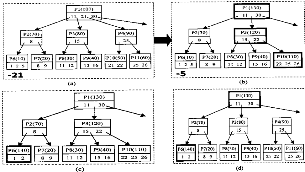
(그림 5) 삭제 연산에 의한 B-트리 구조 변경의 예
