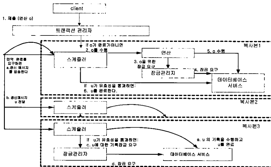
(그림 4) 낙관적인 방법을 적용한 갱신 트랜잭션 처리단계
