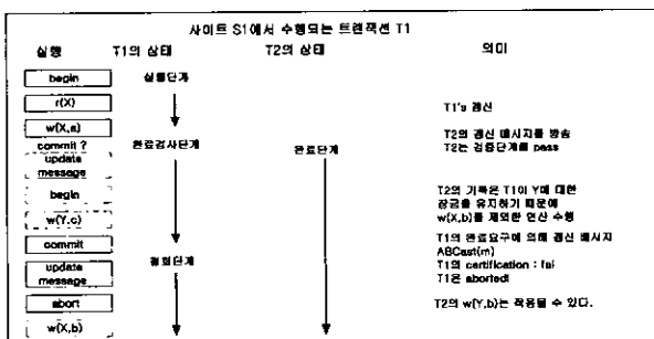
(그림 6) 사이트 S1에서 수행되는 트랜잭션 T1
