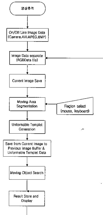
(그림 13) 부분 외곽선 정보를 이용한 이동물체 추적 알고리즘에 대한 순서도
