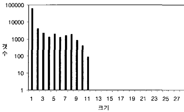
(그림 6) (그림 5)의 이동벡터 크기 히스토그램
