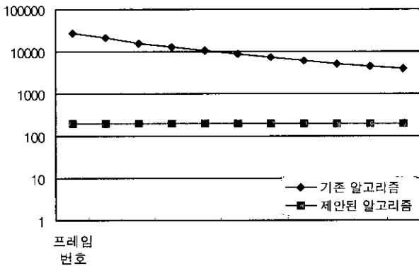
(그림 28) 기존 알고리즘과 제안된 알고리즘의 연산량 비교
