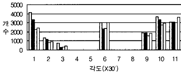
(그림 25) 이동벡터 각도히스토그램
