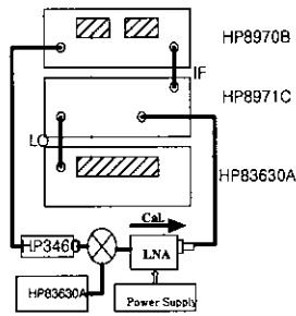
그림 3. 잡음지수 측정용 위한 구성도
