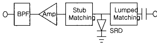
그림 10. 주파수 체배기의 구조도
