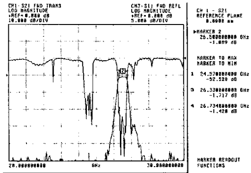
그림 22. 듀플렉서의 RX 필터부의 삽입손실 특성
