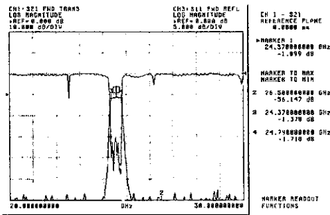
그림 19. TX 필터의 삽입손실 특성
