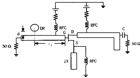
그림 9. 입력 회로에 유전체 공진기를 사용한 직렬 케환형 FET 발전기
