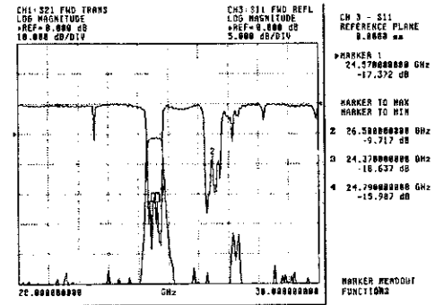
그림 21. 듀플렉서의 TX 필터부의 반사손실 특성
