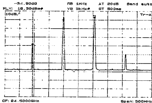
그림 8. SSPA 혼 변조 왜곡(IMD)의 특성
