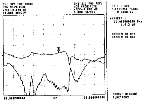
그림 4. 저잡음 증폭기의 이득 특성
