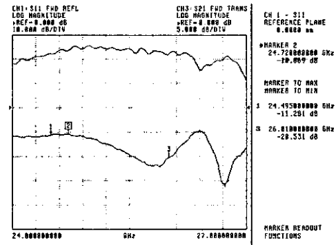
그림 5. 저잡음 증폭기의 반사 특성
