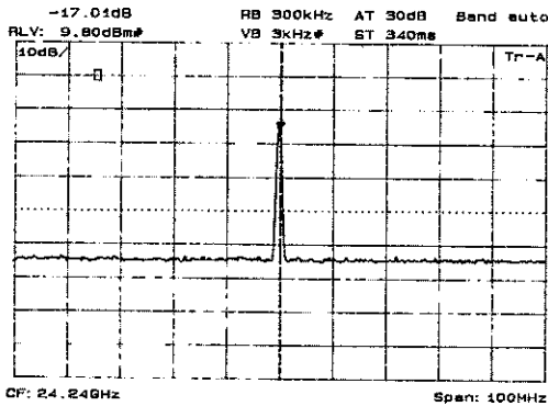
그림 14. 상향용 혼합기의 변환손실 특성결과
