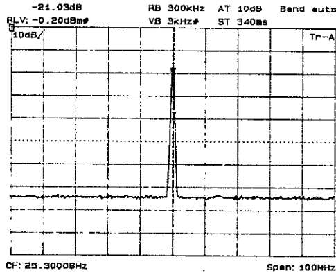
그림 13. 상향용 혼합기의 LO-RF 격리도 특성결과 @ PLO = 0dBm
