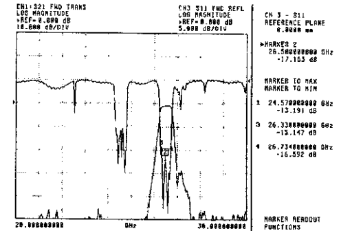
그림 23. 듀플렉서의 RX 필터부의 반사손실 특성
