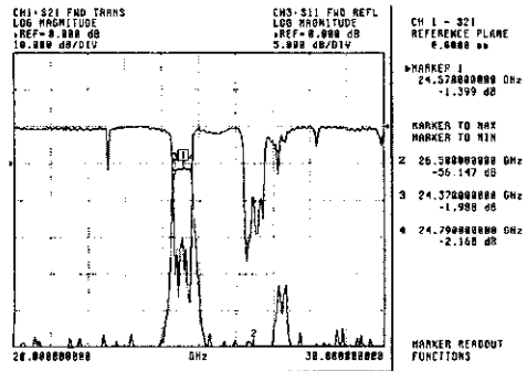
그림 20. 듀플렉서의 TX필터부의 삽입손실 특성
