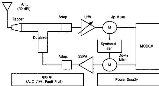
그림 2. LMDS 트랜시버의 구조도
