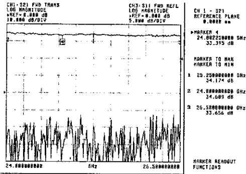
그림 6. SSPA의 이득 특성
