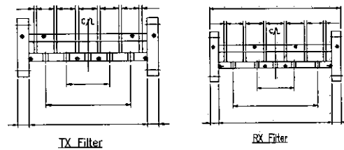
그림 16. 설계된 대칭적 유도성 창을 이용한 대역통과 필터
