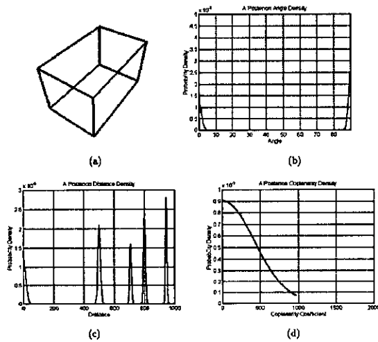
그림 6. 직육면체 모델에 대한 각 속성의 잠음 모델링 결과 (a) 직육면체 모델 (b) 각도 속성의 확률 밀도 함수의 조합 (c) 거리 속성의 확률 밀도 함수의 조합 (d) 동일 평면성 속성의 확률 밀도 함수
