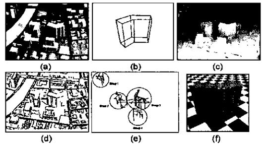
그림 12. 실험결과 (a) 입력 밝기 영상 (b) 3-D 카드 모델 (c) 추정된 거리 영상 (d) 직선 특징 (e) 그룹핑 결과 (f) 복원된 3차원 건물 모델
