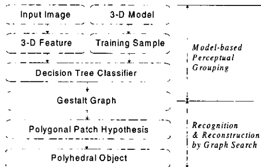
그림 1. 본 논문에서 제안하는 알고리즘의 블록선도
