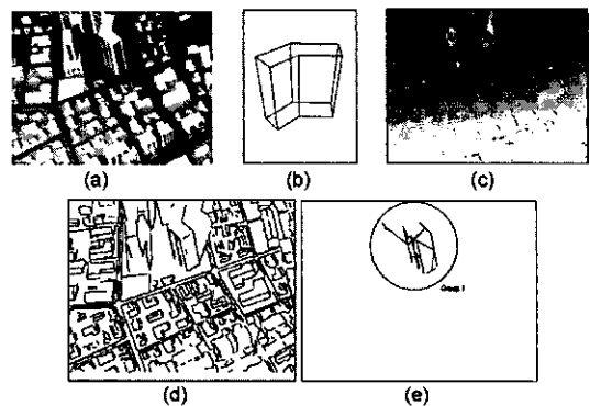
그림 13. 실험결과 (a) 입력 밝기 영상 (b) 3-D 카드 모델 (c) 추정된 거리 영상 (d) 직선 특징 (e) 그룹핑 결과
