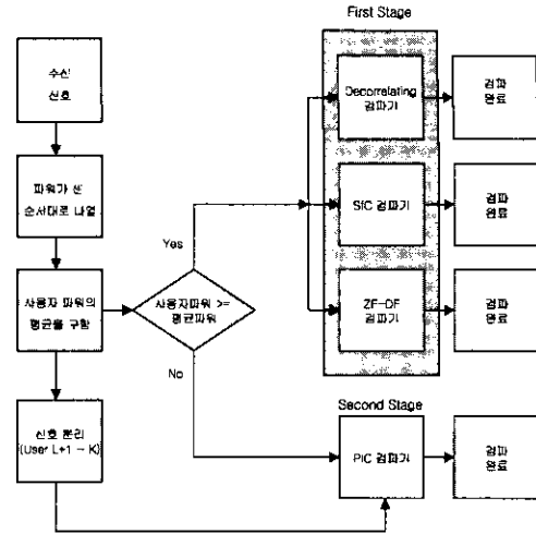
그림 1. 하이브리드 다중 사용자 알고리즘의 순서도
