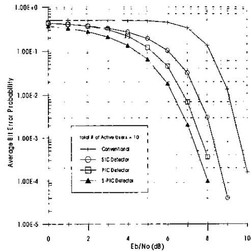
그림 3. S-PIC 검파기의 성능비교
