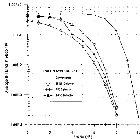
그림 4. Z-PIC 검파기의 성능비교
