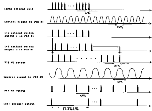
그림 3. 96년 발표된 ULPHA 스위치용 광 셀 역압축기의 역압축 타이밍도
