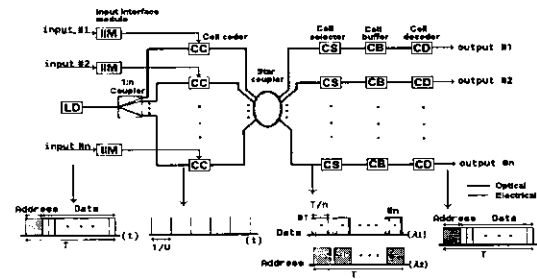
그림 1. ULPHA 스위치의 블록도
