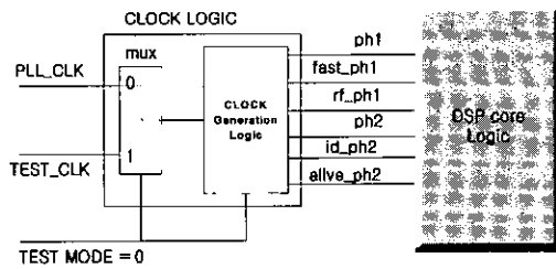
그림 5. Embedded clock controller
