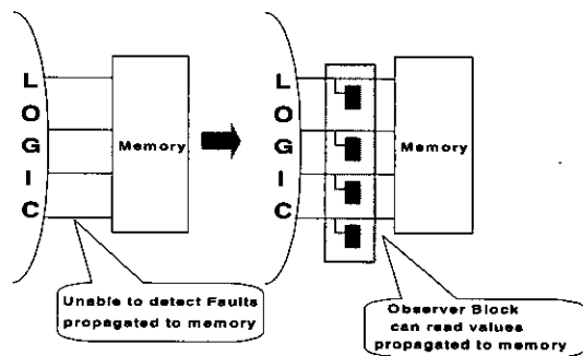
그림 10. 관찰도를 높이기 위한 F/F 추가
