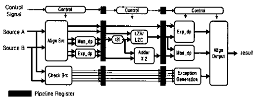
그림 6. FALU의 상위 서브블럭
