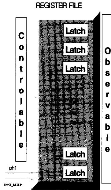
그림 9. 레지스터파일의 테스트용이설계
