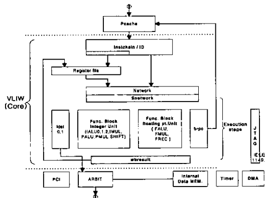
그림 1. FLOVA의 구조
