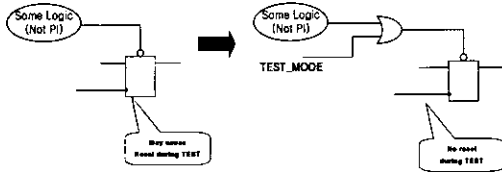
그림 11. 비동기리셋으로 부터의 보호
