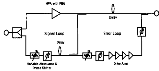
그림 5. 전방급전 전력증폭기 회로도
