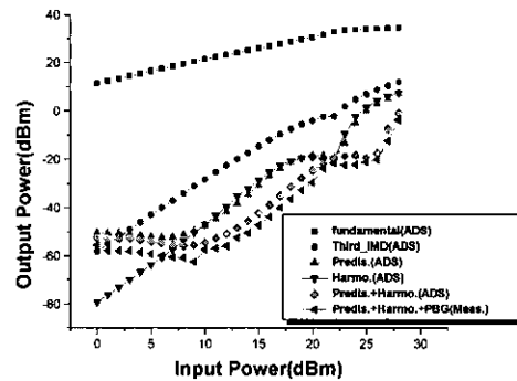
그림 2. 시뮬레이션 및 측정된 주 증폭기의 출력 및 IMD특성
