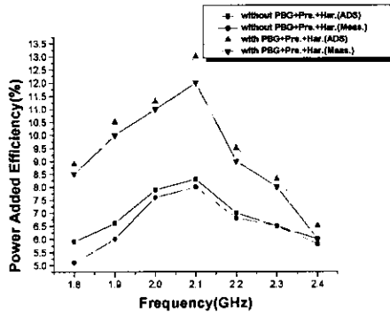
그림 3. 전방급전 전력증폭기의 효율
