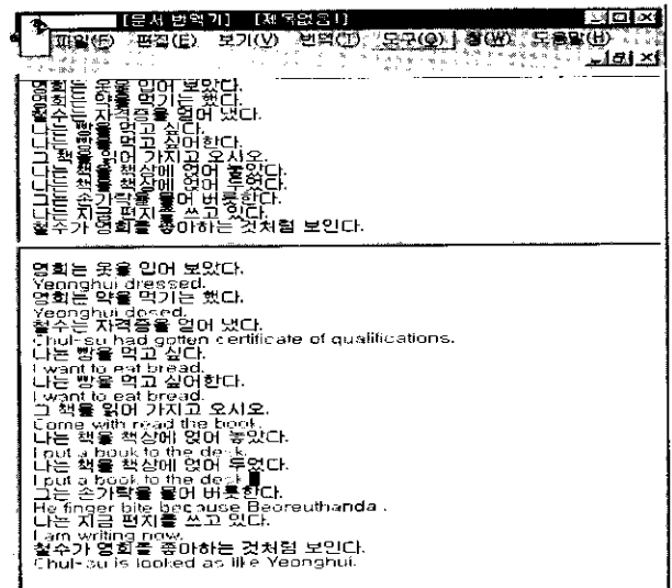
(그림 4) 상용 자동 번역시스템에서의 보조동사처리의 예
