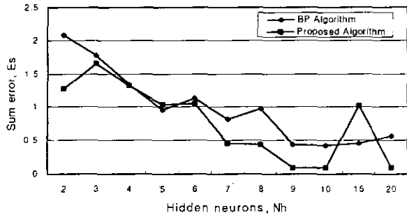
(그림 3) 은닉층 뉴런수 Nh에 따른 합오차 Es의 변화
