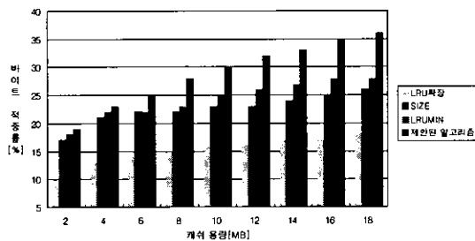
(그림 7) 바이트 적중률 비교(서버 2)
