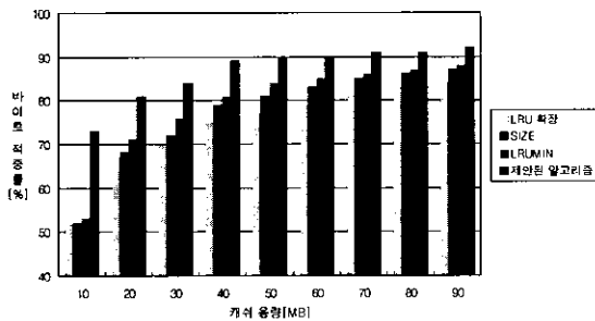
(그림 6) 바이트 적중률 비교(서버 1)
