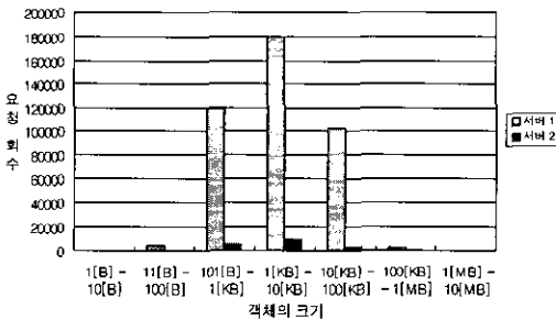
(그림 2) 객체 크기별 요청 회수
