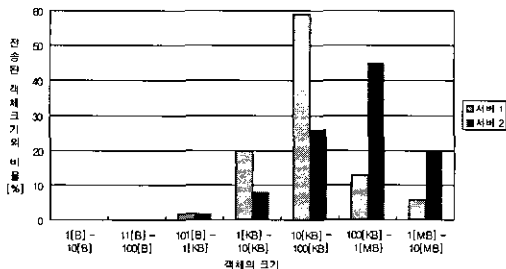
(그림 3) 객체 크기별 총전송량 비율
