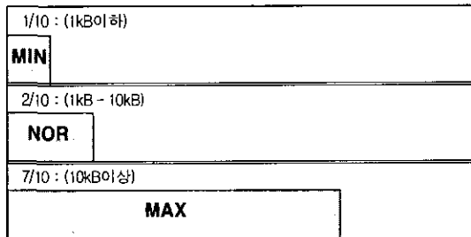
(그림 1) 캐쉬 메모리의 분할 구조
