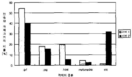
(그림 5) 객체 포맷별 총전송량 비율
