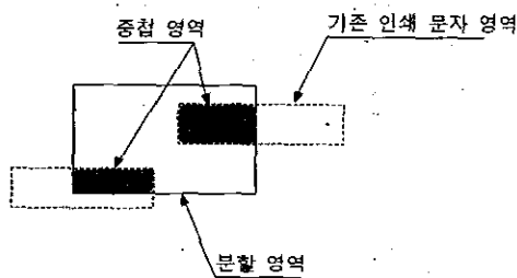
(그림 7) 분할 영역과 기존 인쇄 문자 영역의 중첩
