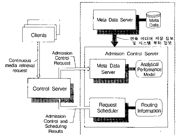
(그림 2) CCMSS 시스템의 승인 제어 모델
