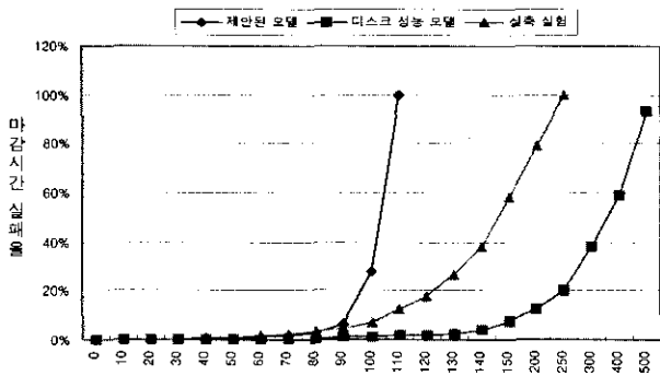
(그림 4) 제안된 승인 제어 기법에 의한 최대 허용 가능한 검색 요구 수
