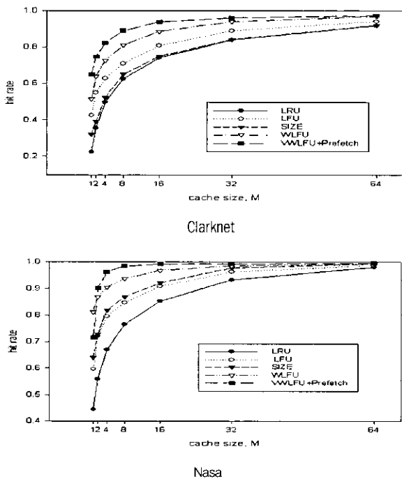
(그림 10) 선인출 기법과 기존의 정책과 비교(히트율)
