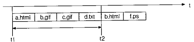
(그림 6) HTML문서의 요청과 그 외 파일들에 대한 요청열
