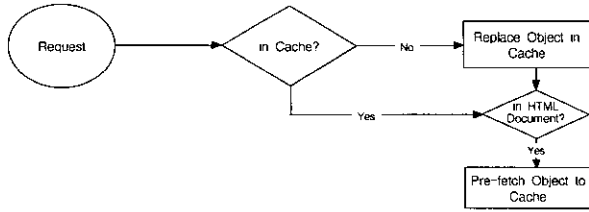
(그림 9) 선인출 알고리즘
