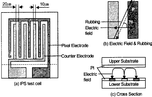
그림 1. IPS 셀의 구조.
