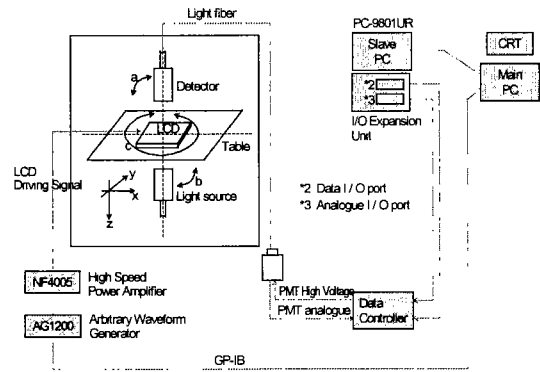
그림 2. V-T 히스테리시스 측정 시스템.
