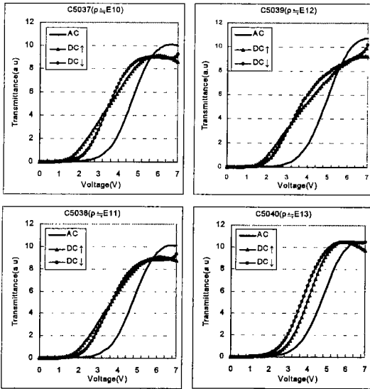
그림 4. 불소계 액정의 비저항 별 V-T 히스테리시스 특성.
