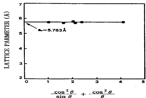
그림 4. CuInSe 2 의 격자 상수 a 0 .
