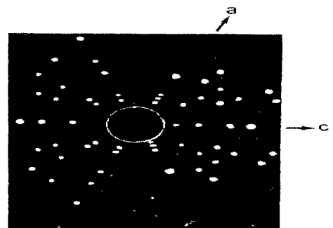
그림 8. 배면 반사법으로 측정된 (112)면의 Laue 무늬. Fig. 8. Back-reflection Laue patterns for the (112) planes.
