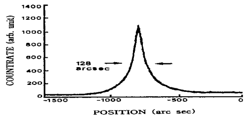
그림 7. CuInSe 2 단결정 박막의 이중 결정 X-선요동곡선. Fig. 7. Double crystal X-ray rocking curve of CuInSe 2 single crystal thin film.
