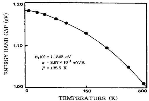
그림 15. CuInSe 2 단결정 박막의 온도에 따른 띠간격 (실선은 Varshni 방정식을 나타냄). Fig. 15. Temperature dependence of the energy gap for CuInSe 2 single crystal thin film (The solid line represents the fit to the Varshni equation).
