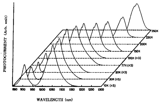
그림 13. CuInSe 2 단결정 박막의 광전류 스펙트럼.
