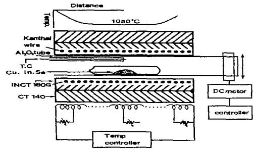
그림 1. CuInSe_2 다결정 합성 수평 전기로. Fig. 1. Horizontal electric furnace for synthesizing CuInSe_2 polycrystal.
