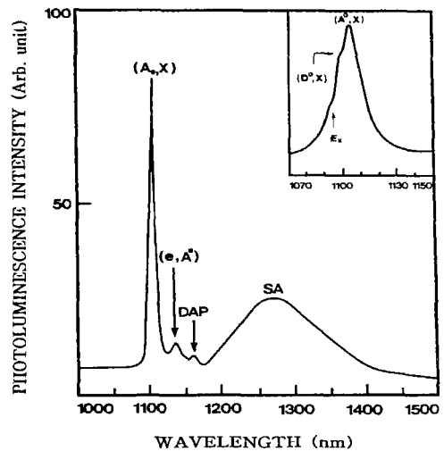
그림 16. CuInSe 2 단결정 박막의 10K에서 광발광 스펙트럼.
