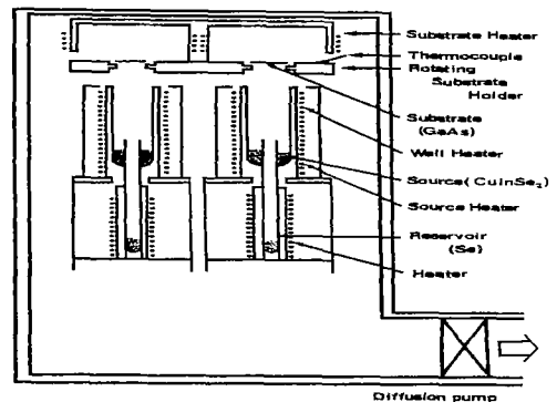
그림 2. HWE 장치의 개략도. Fig. 2. Schematic diagram of the hot wall epitaxy system.
