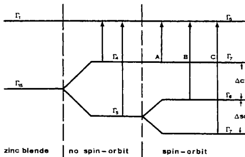
그림 14. CuInSe 2 에너지 준위의 미세구조. Fig. 14. Fine structure for energy level of CuInSe 2 .
