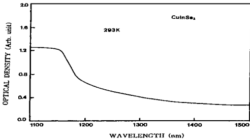
그림 11. CuInSe 2 단결정 박막의 광흡수 스펙트럼.
