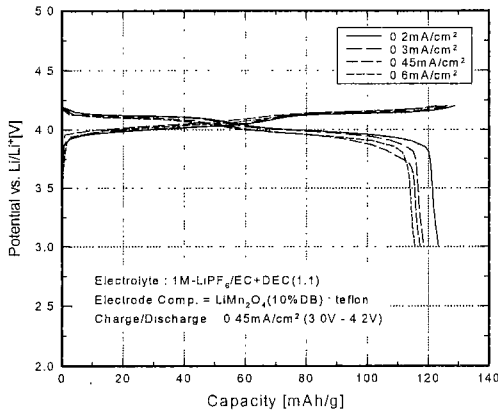
그림 3. 전류밀도를 변화한 경우의 스피넬 LiMn 2 O 4 의 충방전 용량.
