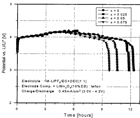
그림 5. 리튬 과량(0≤x≤0.075)을 변화하여 제조한 스피넬 Li_{1+x}Mn_2O_4 의 1회 사이클의 용량곡선.
