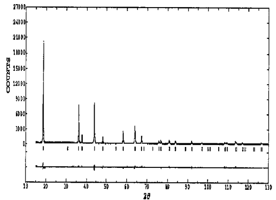
그림 2. 750^\circ\text{C} 에서 제조한 \text{LiMn}_2\text{O}_4 시료의 리트벨트 정밀화한 경우의 X-선 회절 패턴.
