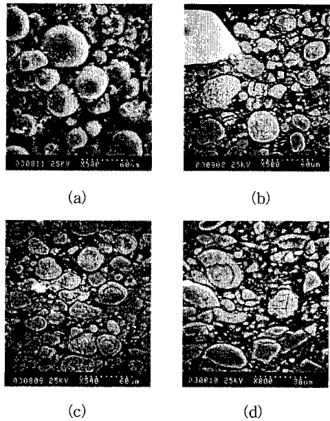
그림 7. 리튬 양을 변화하여 제조한 Li_{1+x}Mn_2O_4 의 SEM 사진.
