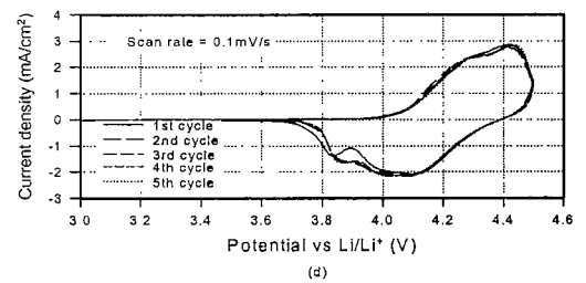
그림 4. Li/Li 1-x Mn 2 O 4 전지의 순환전위 전류곡선. (a) LiMn 2 O 4 , (b) Li 1.025 Mn 2 O 4 , (c) Li 1.05 Mn 2 O 4 , and (d) Li 1.075 Mn 2 O 4
