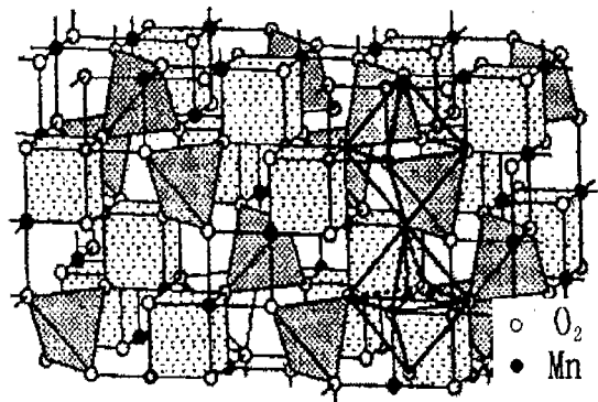
그림 1. 스피넬 LiMn 2 O 4 의 결정 구조. Fig. 1. Crystal structure of spinel LiMn 2 O 4 .
