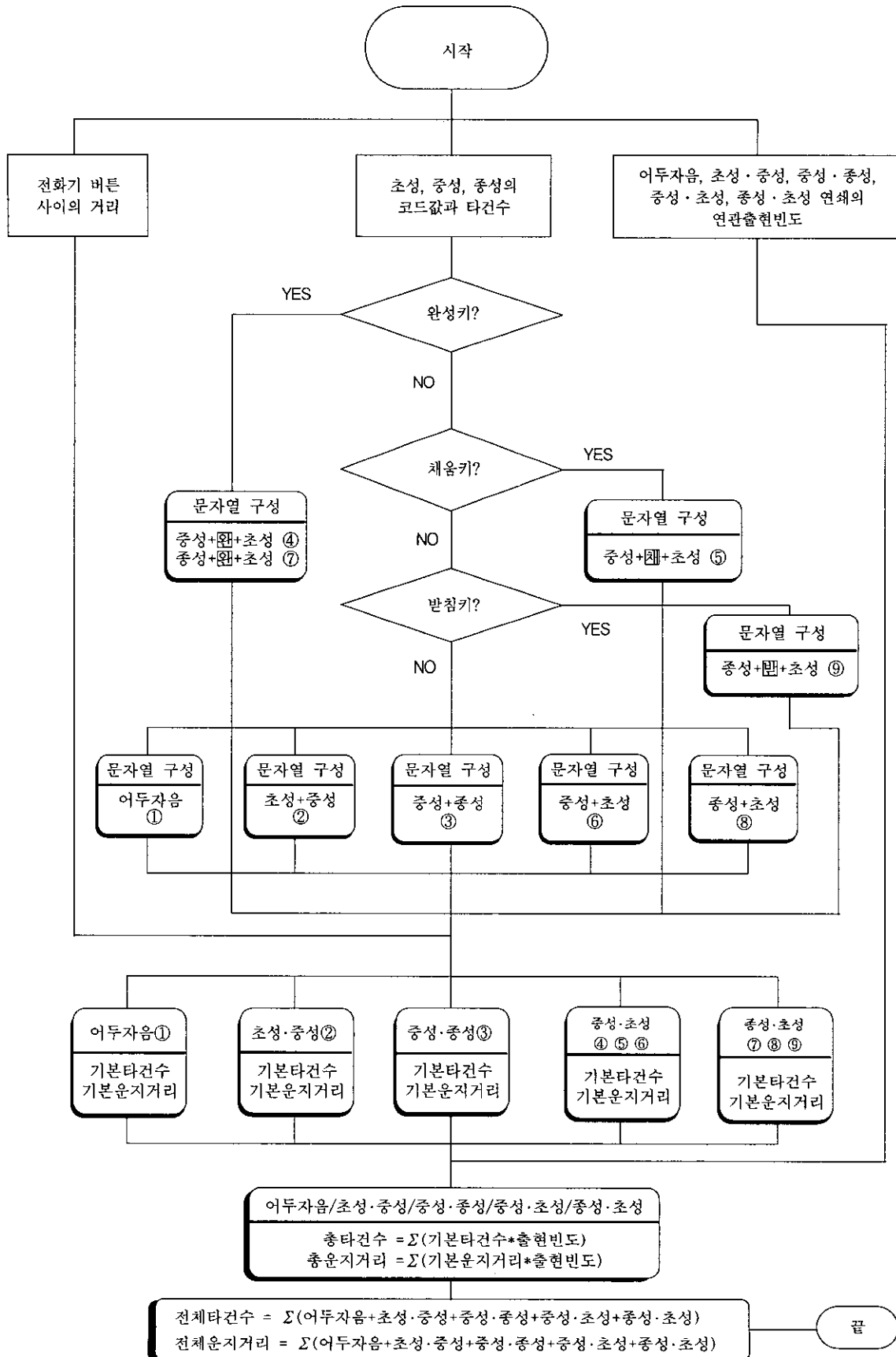
(그림 1) 전화기 한글자판의 타건수와 운지거리 계산 순서도
