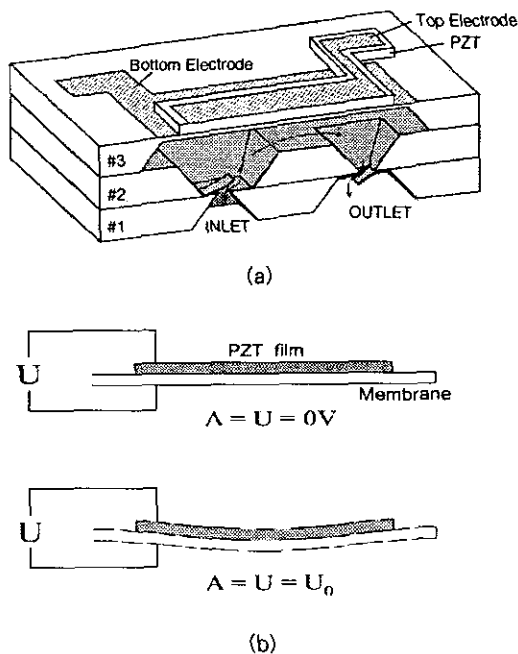
그림 1. (a) PZT 구동 다이아프램 펌프와 (b) PZT 구동 다이아프램의 구동원리
