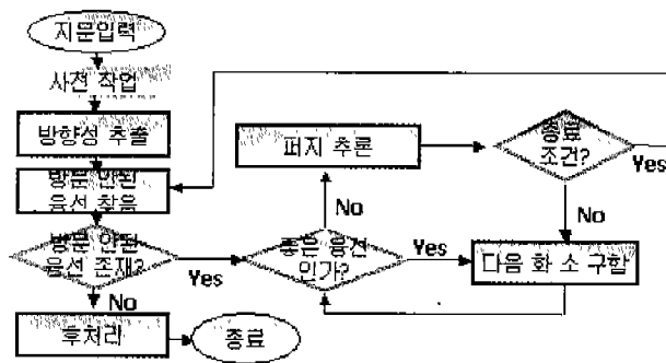
그림 4. 제안된 방법의 알고리즘 흐름도 Fig 4. Flow Chart of the proposed method
