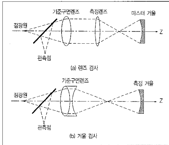
그림 5 mirror 측정을 위한 간섭계
