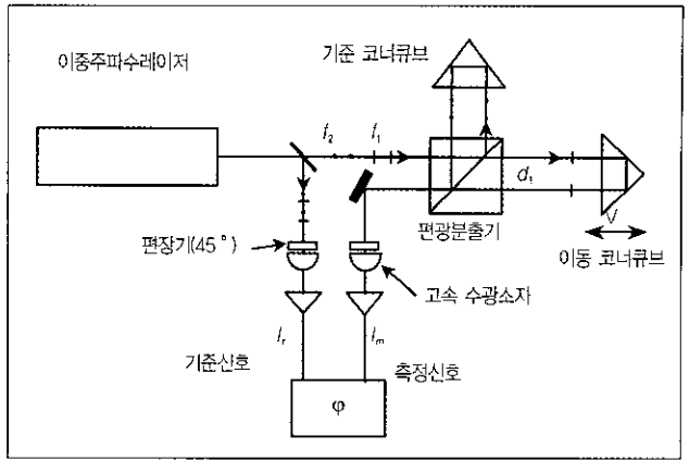
그림 2 헤테로다인 간섭계
