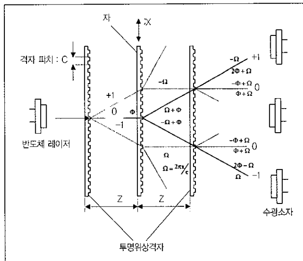
그림 4 Heidenhain식 광학 스케일의 개념도
