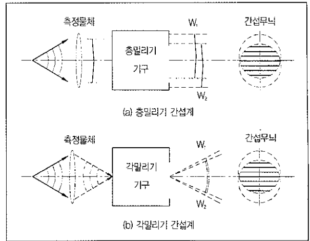
그림 6 총밀립 간섭계의 구성도
