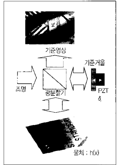
그림 8 광위상 간섭계의 개념도
