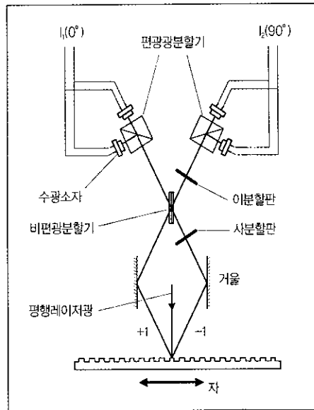
그림 3 편광을 이용한 광학스케일의 개념도
