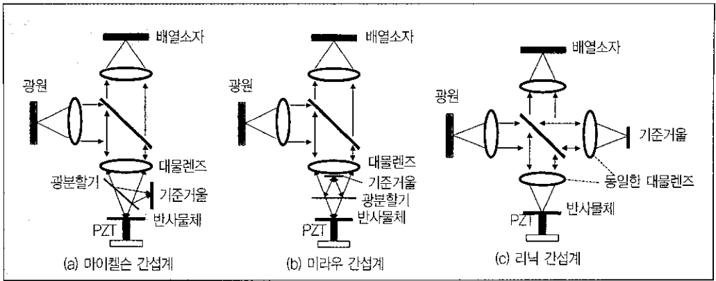
그림 7 간섭계의 개념도 그림
