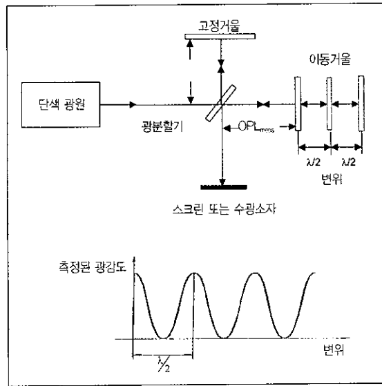
그림 1 마이켈슨 간섭계
