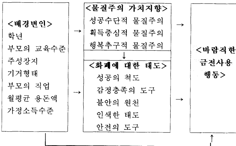
<그림 1> 연구모형
