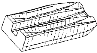
그림 9. Dual AIR의 선저 형상
