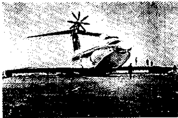
그림 11. WIG(러시아의 ORLYONOK)
