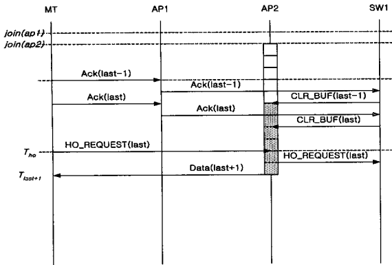
(그림 10) positive ack 핸드오프 절차
