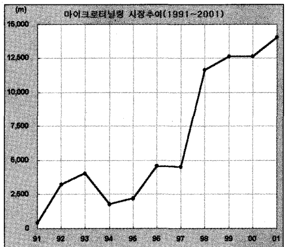
그림 1. 국내의 마이크로터널링 공법에 의한 건설시장의 추이
