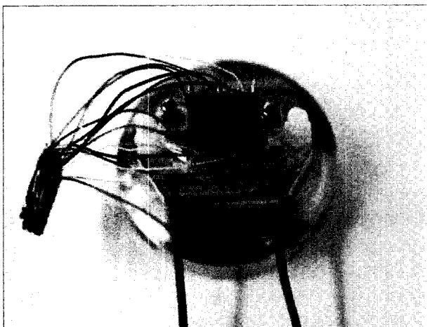
그림 2. 카메라 헤드의 내부에 부착된 TC-245 CCD
