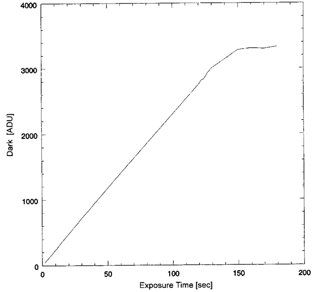
그림 5. 유효 반응 범위(Dynamic Range) 그래프.
