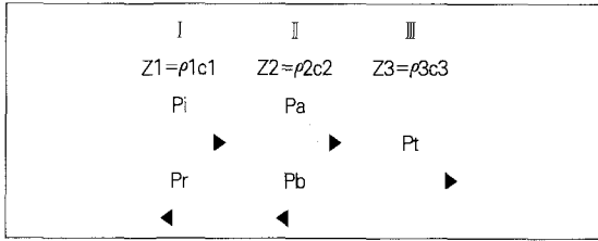
그림 2. 매질 경계에서의 초음파의 투과 및 반사
