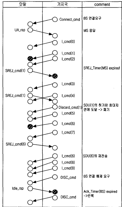
(그림 1) 제안한 ARQ 프로토콜의 동작 예
