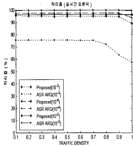
(그림 5) 실시간 트래픽의 처리율
