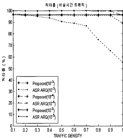
(그림 7) 비실시간 트래픽의 처리율
