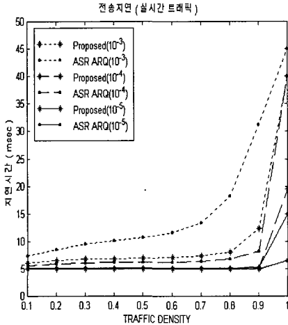
(그림 4) 실시간 트래픽의 전송지연
