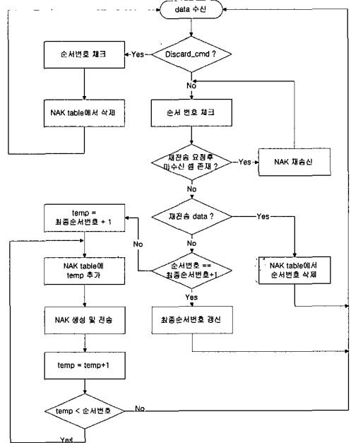
(그림 3) 수신단 동작절차
