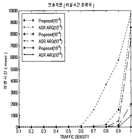
(그림 6) 비실시간 트래픽의 전송지연
