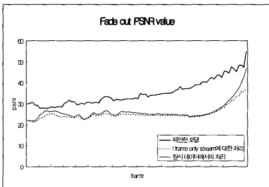
그림 17 페이드 아웃 효과에서의 화질 비교
