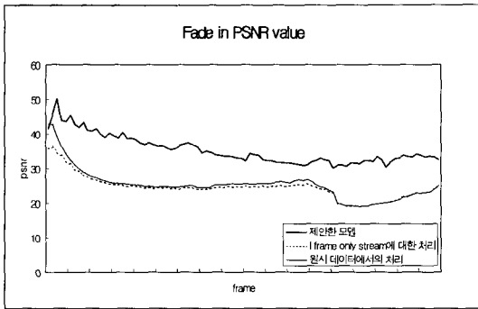
그림 16 페이드 인 효과에서의 화질 비교
