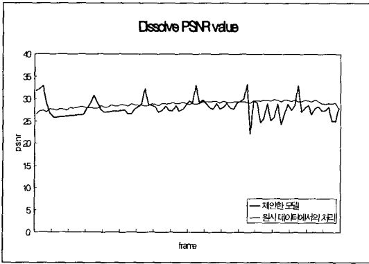
그림 19 움직임이 적은 스트림간 디절브 효과에서의 화질 비교
