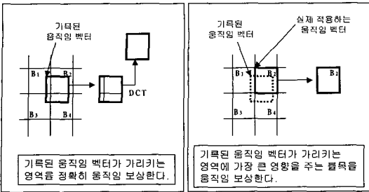
(a) 기존의 움직임 보상 방법 (b) 제안한 움직임 보상 방법 그림 7 움직임 보상 방법의 비교
