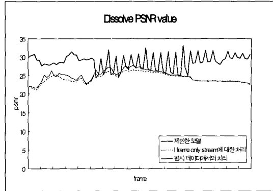
그림 18 디절브 효과에서의 화질 비교
