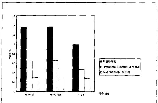
그림 15 각 적용 방법 별 처리 속도의 비교
