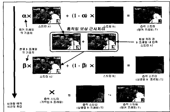
그림 8 B-프레임에 대한 처리 방법
