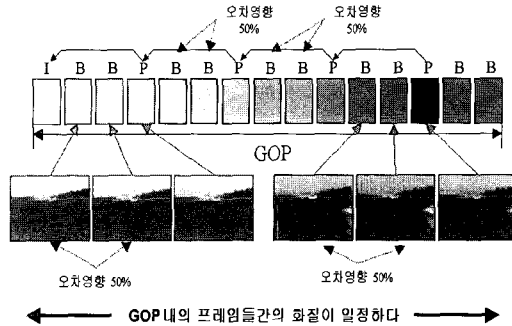
GOP내의 프레임들간의 화질이 일정하다
