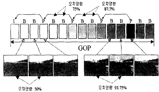
GOP내 프레임의 화질은 처음에서 뒤로 갈수록 악화된다
