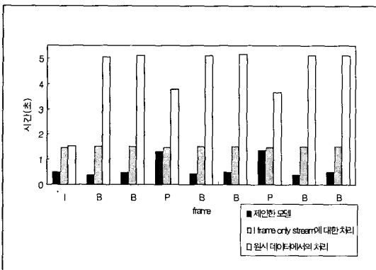
그림 14 프레임 형식 별 생성 시간
