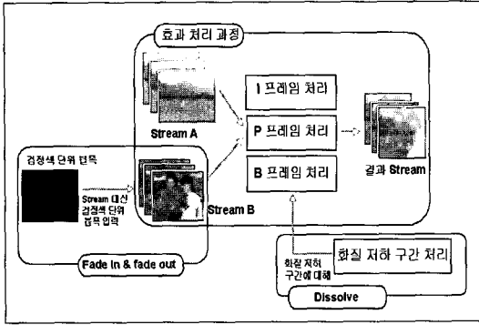
그림 4 전체 전환 효과 처리 과정
