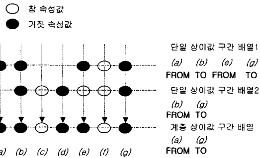
그림 2 구간 배열의 병합 과정
