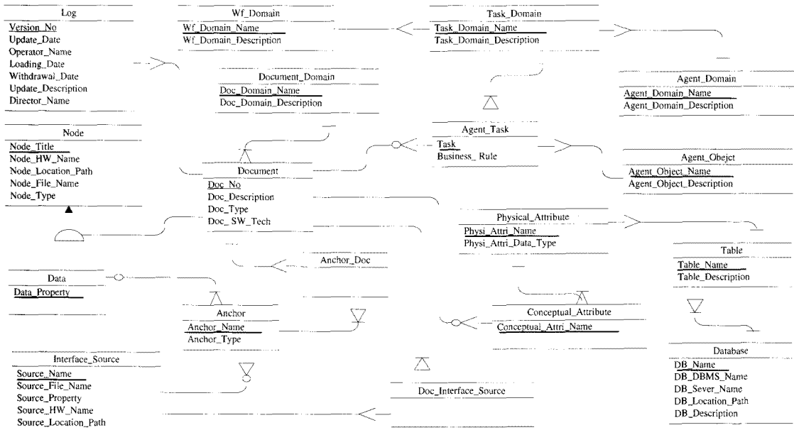
<그림 12> HyDoMIS의 데이터베이스 스키마
