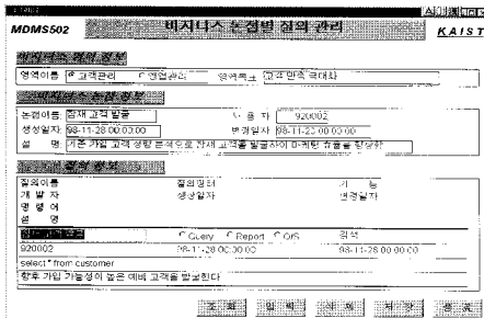
(그림 4-11) 비즈니스 논점별 질의 관리 화면 (비즈니스 계층)
