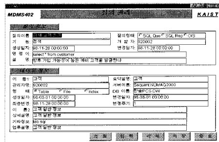
<그림 4-10> 질의 관리 화면 (사용자 탐험 계층)
