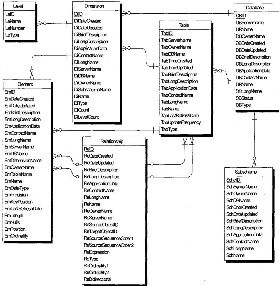
<그림 3-2> MDIS 표준 기반 메타데이터 스키마
