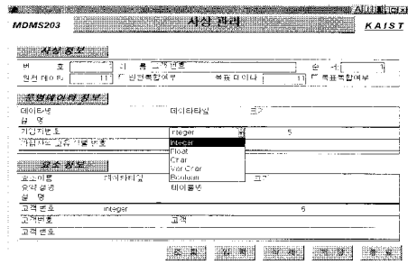
<그림 4-6> 사상 관리 화면 (적용 계층)
